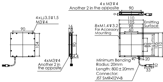
7.OPT-FL110110
