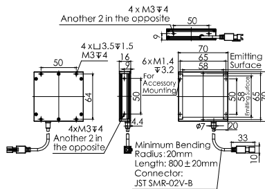
5.OPT-FL7070
