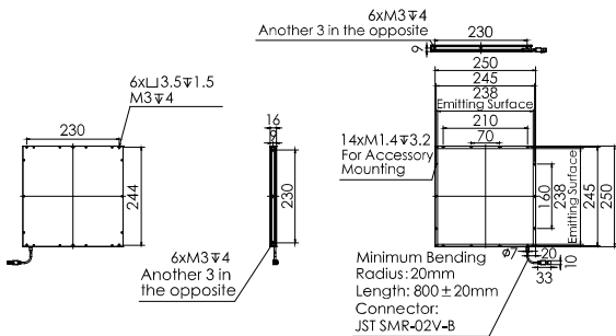
13.OPT-FL250250
