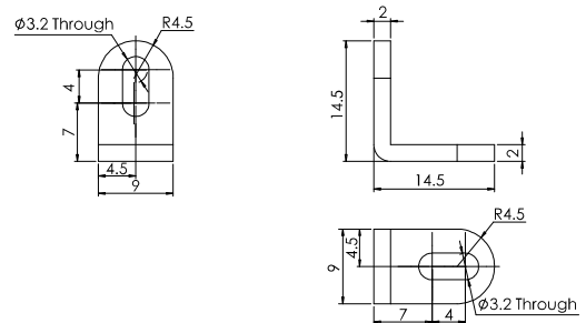
14.OPT-PRIN1515
