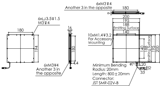
11.OPT-FL200200
