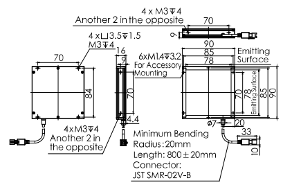
6.OPT-FL9090
