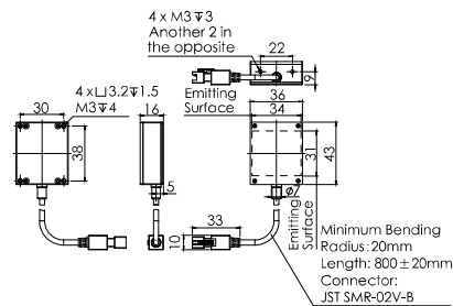
2.OPT-FL4336
