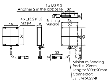
4.OPT-FL6254
