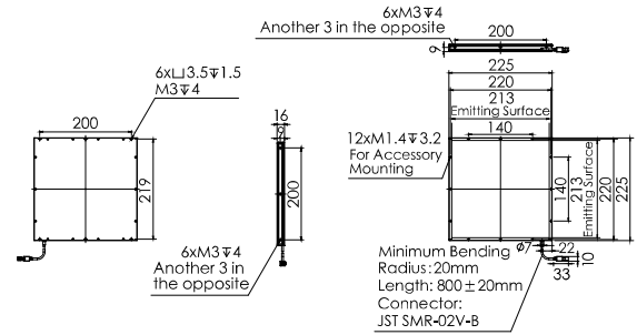
12.OPT-FL225225
