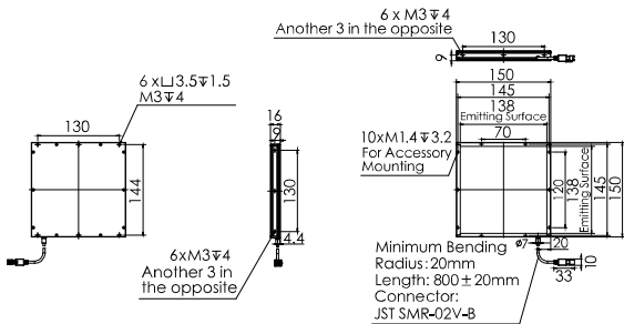
9.OPT-FL150150
