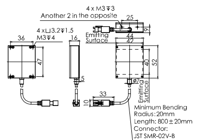
3.OPT-FL5244
